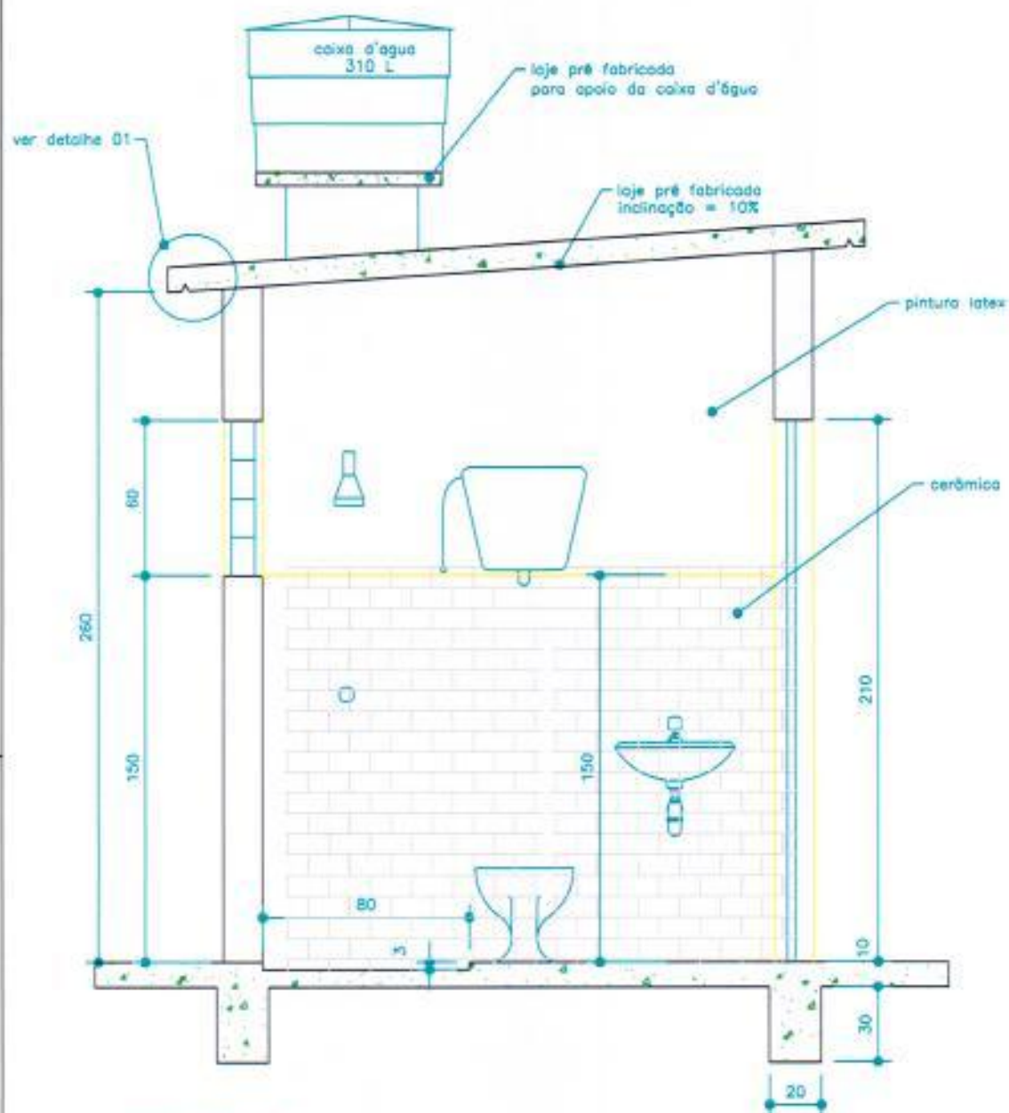
CORTE BB
